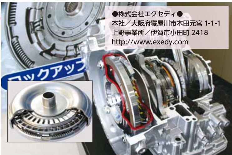
上野事業所で製造しているトルクコンバータ(枠内)とトルクコンバータを搭載したATミッション
